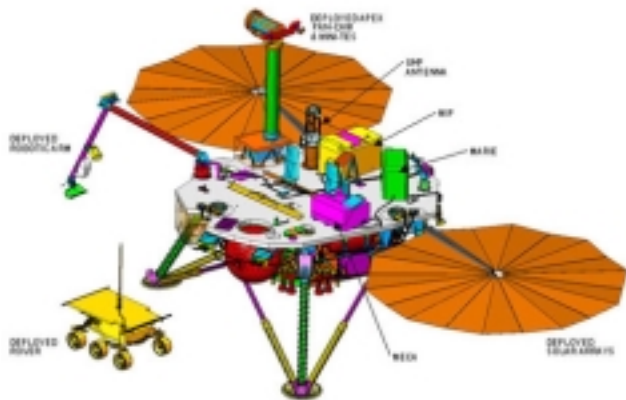
Figure 1 - Mars 2001 Lander
